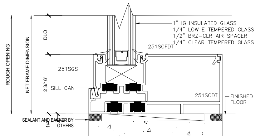
⑤ SILL CAN (@SIDELITE) STOREFRONT SIDELITE SCALE: 1'-0" = 1'-0"
