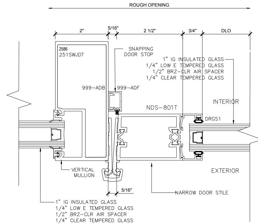
① SIDELITE & JAMB (@STOREFRONT PAIR DOORS) HINGE: GEAR HINGE SCALE: 1'-0"=1'-0"
