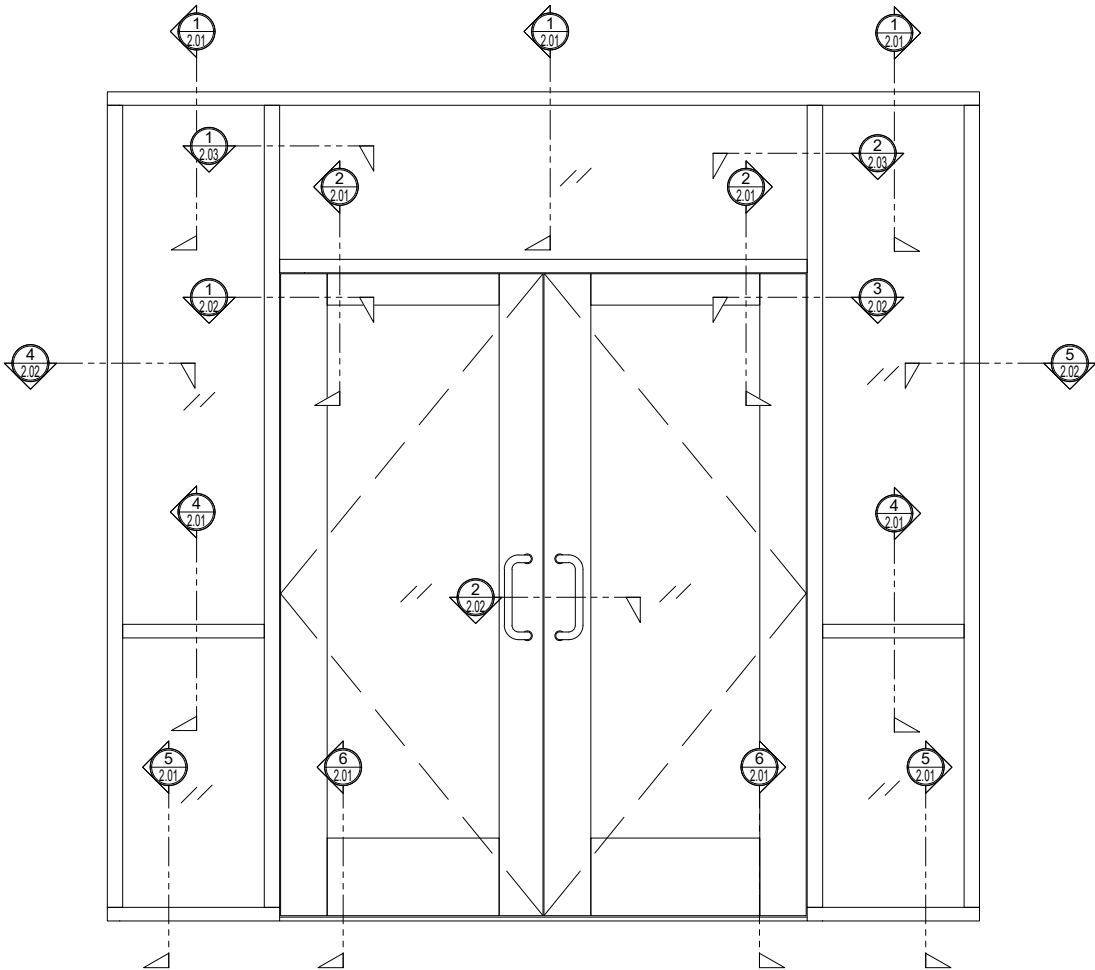
③ ELEVATION STOREFRONT (PAIR)
