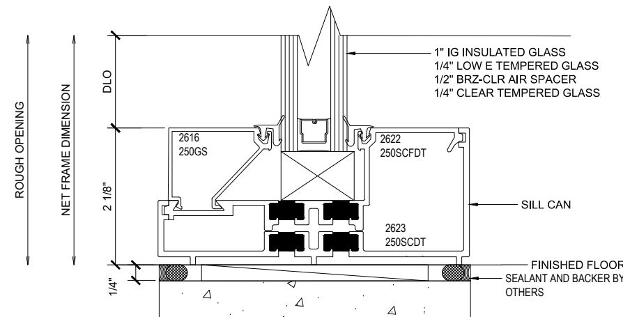
⑤ SILL CAN (@SIDELITE) STOREFRONT SIDELITE SCALE: 1'-0" = 1'-0"
