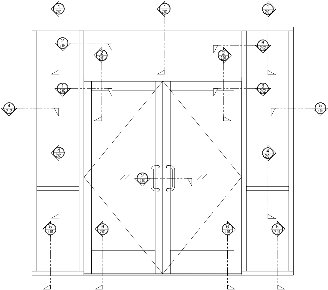
3 ELEVATION STOREFRONT (PAIR)
