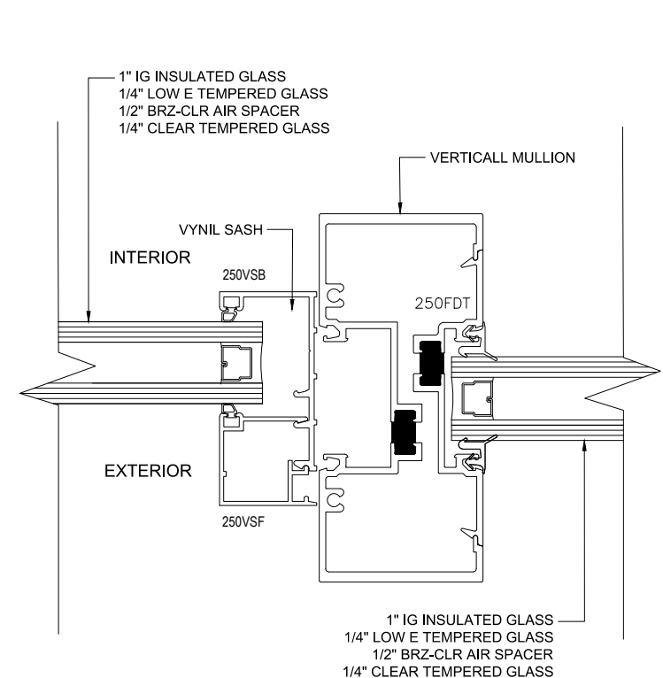
⑥ TRANSOM & SIDELITE (@VYNIL SASH)
