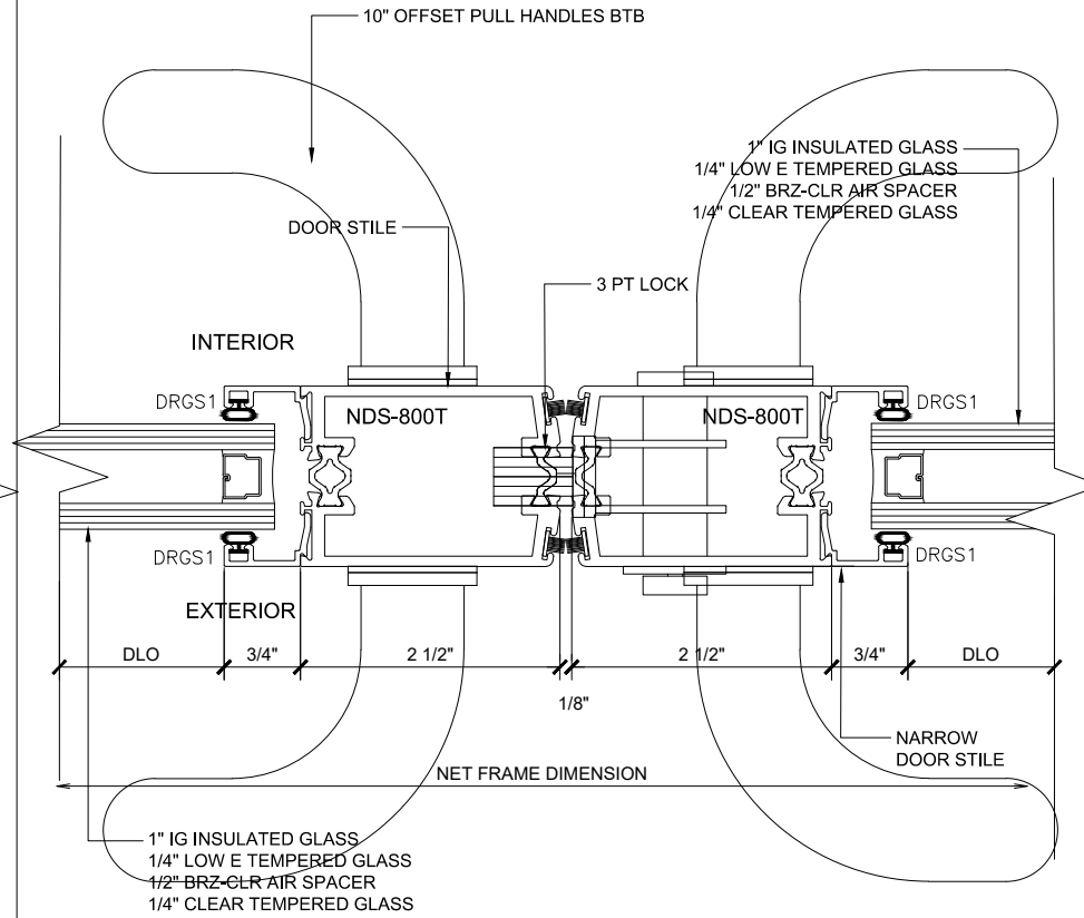
② DOOR STILES (@DOOR)
