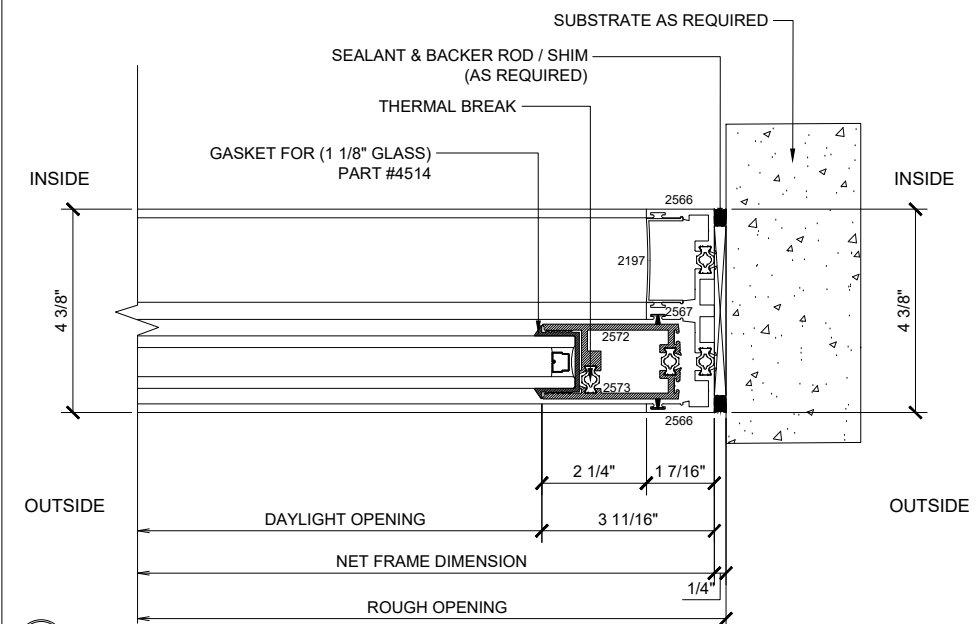
⑥ JAMB
