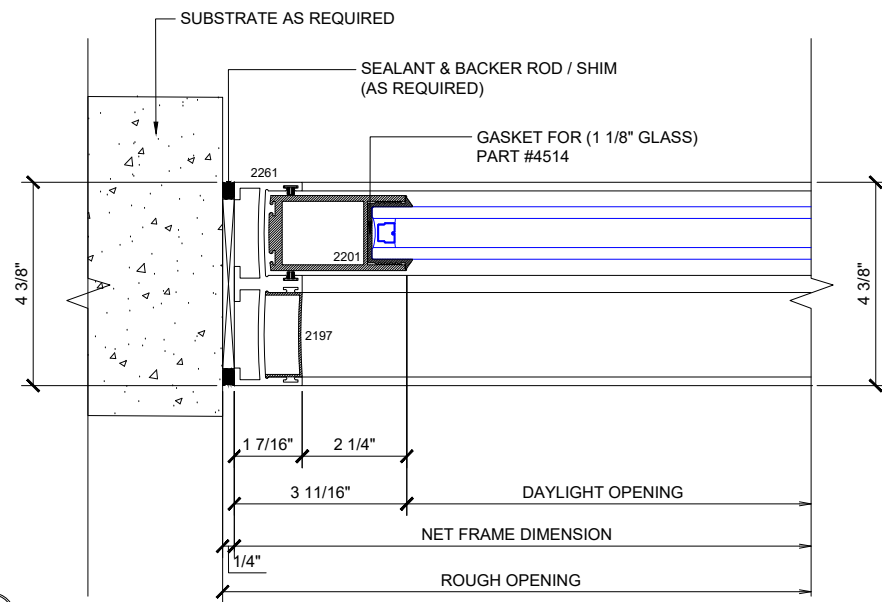
① JAMB
