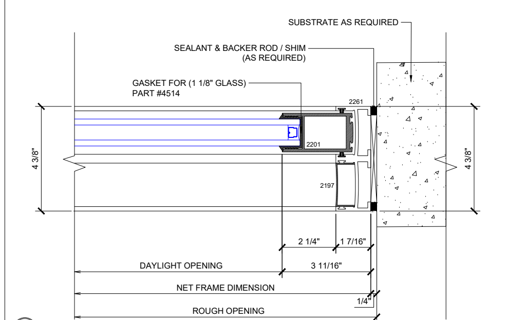
⑥ JAMB
