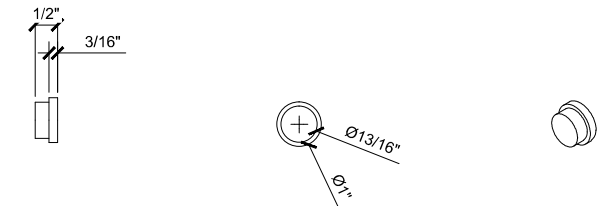
(G) PLECAP RUBY END CAPS RUBY SLIDING DOORS (OXO) SCALE: 6"=1'-0"
