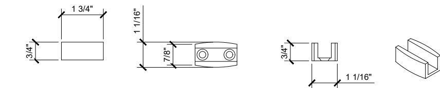
© TIFFANY SLIDING DOOR GUIDE
