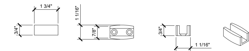
③ TIFFANY SLIDING DOOR GUIDE
