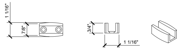
③ TIFFANY SLIDING DOOR GUIDE
