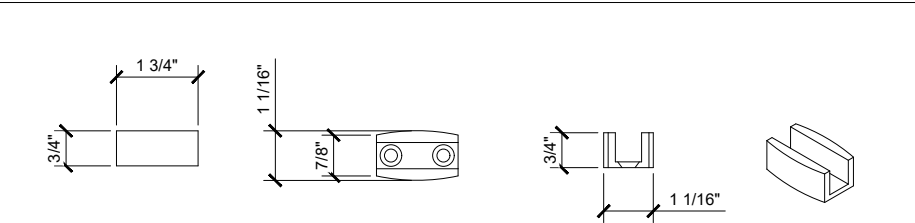
© TIFFANY SLIDING DOOR GUIDE
