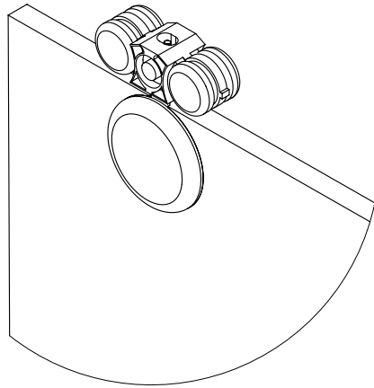
SECTION A-A SLIDING DOOR ROLLER
